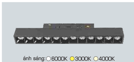
RNC 02 LED 12W - DC 48V 398.000 L222 x W22 x H44 Điện áp: DC 48V Bóng LED SMD 90Lm/W - RA90 Thân đèn: Hợp kim nhôm Góc chiếu: 24°
