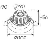
AFC 596 9W 388.000 ĐÈN LED 9W 9.001 - 9.002 - 9.003
