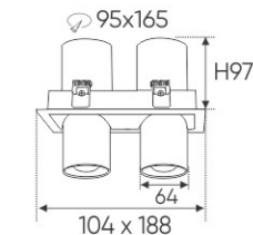
AFC 788/2 12W 1.572.000 ĐÈN LED 12W 12.001 - 12.002 - 12.003
